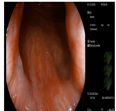
[6]Anal canal
