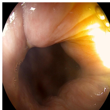
[7]Anal canal
