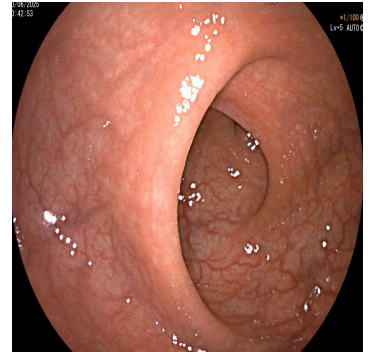
[2]Rectum
