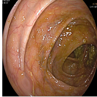
[11] Cecum
