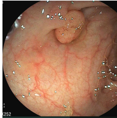
[1]sigmoid
