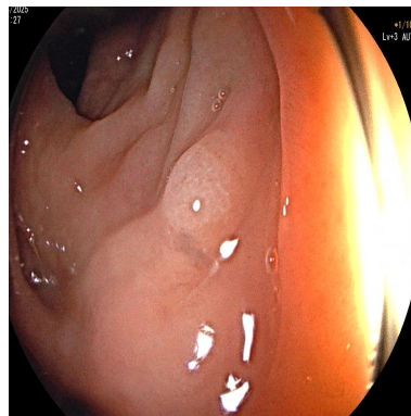
[7]polyp
