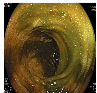
[8]Terminal ileum
