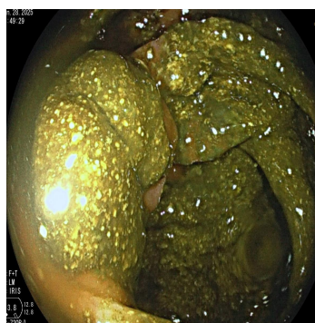
[7]Cecum
