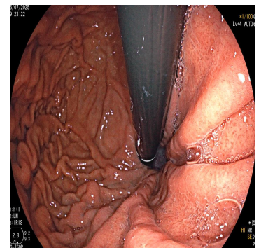
[6]Fundus
